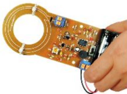
2. 金属探知機
